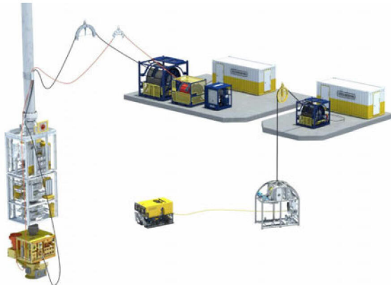
Figur 4: Tradisjonelt IWOCS koblet til en BOP og ventiltre. Til høyre er en ROV (OCEANEERING).
